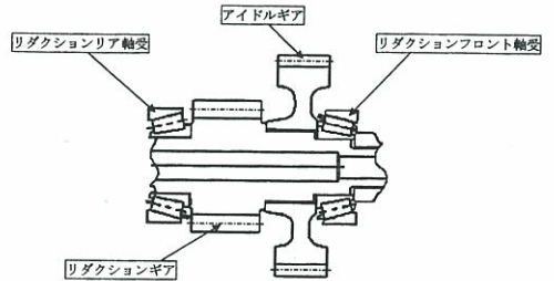
図6 リダクション支持軸受の使用箇所 2)
