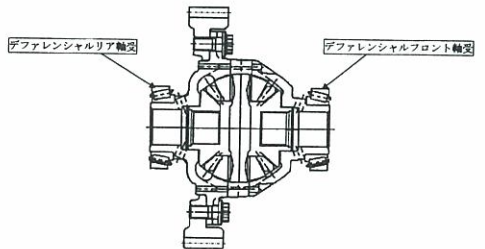
図7 デファレンシャル支持軸受の使用箇所 3)
