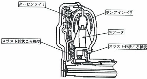
図3 トルクコンバータの構造 2)
