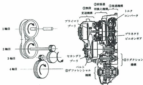
図1 前輪駆動車用ベルト式CVTの構造例 1)
