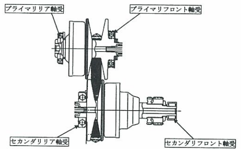
図5 プリー支持軸受の使用箇所 2)
