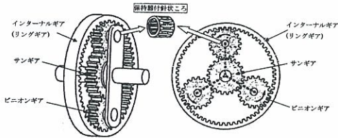
図4 プラネタリの構造 3)
