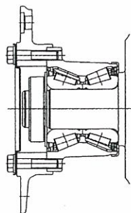
図5 第2世代HURの使用例（従動輪用）
