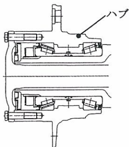
図3 セットライト軸受の使用例
