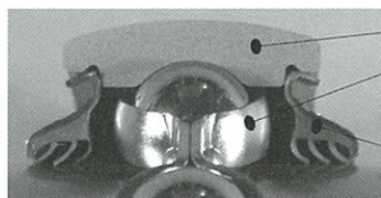
図7 トリプルリップシール付き インサート軸受
