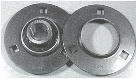
図9 鋼板製フランジタイプ
